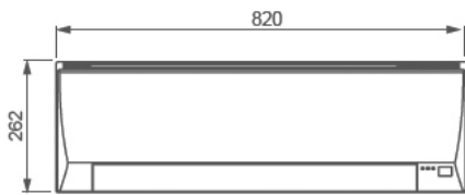
Unidad interior
