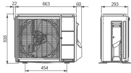
Unidad exterior
